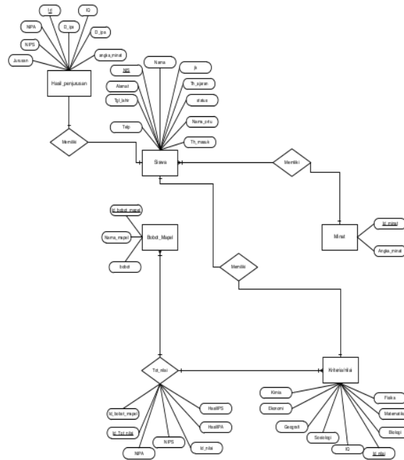
Gambar 7. ERD
