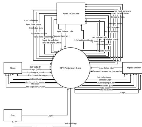
Gambar 1. Diagram Konteks
