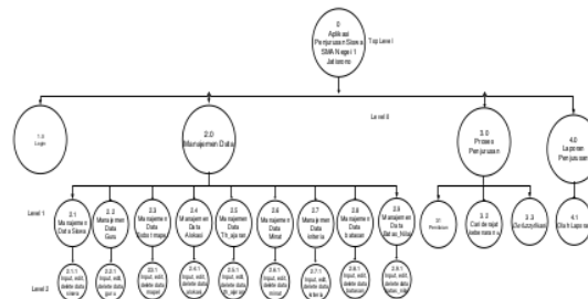
Gambar 2. Diagram Berjenjang
