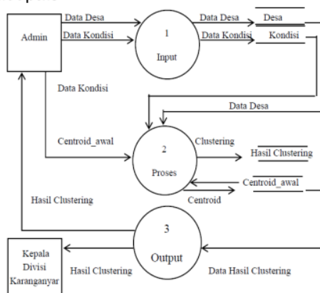
8 Gambar 2. DFD Pamsimas
