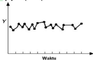
Gambar 1. Pola Data horizontal
