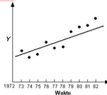
Gambar 4. Pola Data Trend
