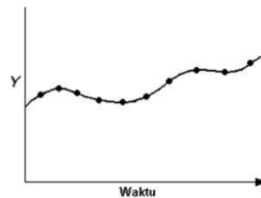
Gambar 3. Pola Data Siklus
