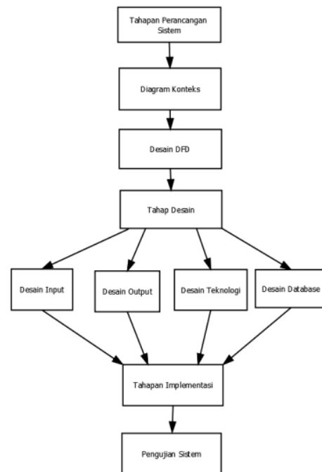
Gambar 5 Diagram Perancangan Sistem
