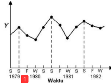
Gambar 2. Pola Data Musiman
