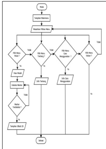
Gambar 5. Flowchart Aplikasi MAR Simulasi jilbab
