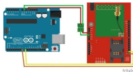
Gambar 5. Rangkaian GSM Shield
