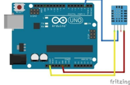
Gambar 3. Rangkaian sensor DHT11
