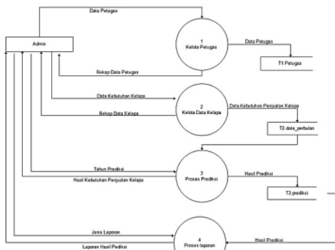
Gambar 2. DFD Level 0 Diagram Alir Perancangan Prediksi
