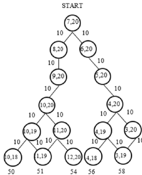
Gambar 8. Perhitungan Langkah 12
