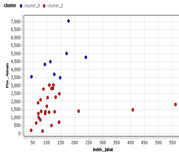
Gambar 4.3. Pengelompokan berdasarkan Jumlah Pos Keamanan dan Indeks Kejahatan
