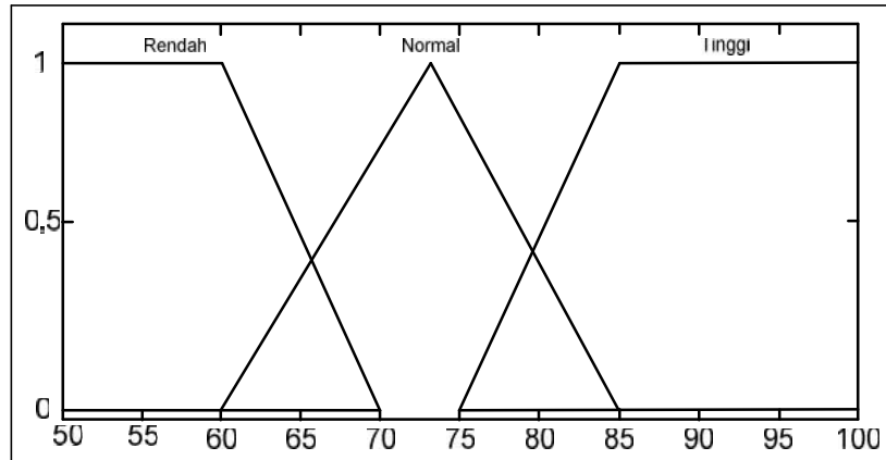
Gambar 4.4. Grafik NIPS
