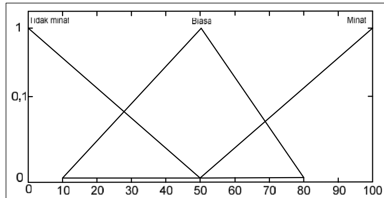
Gambar 4.8. Grafik MINAT
