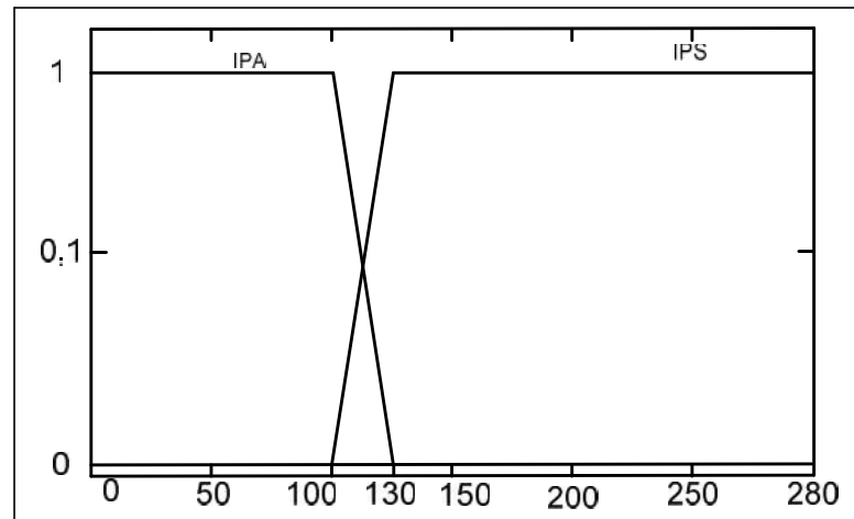
Gambar 4.10. Grafik KAPASITAS
