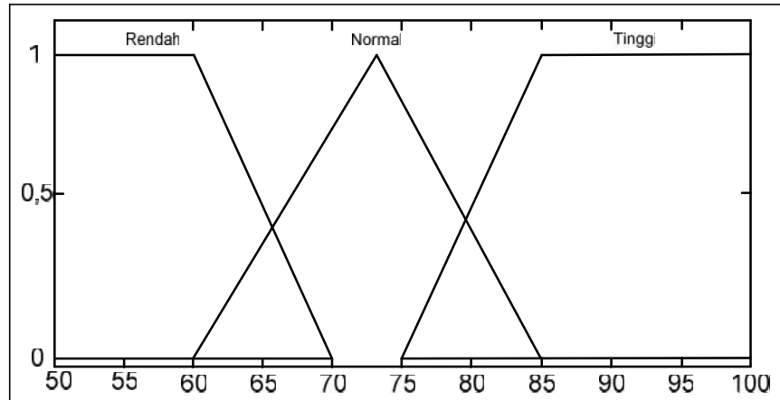
Gambar 4.2. Grafik NIPA
