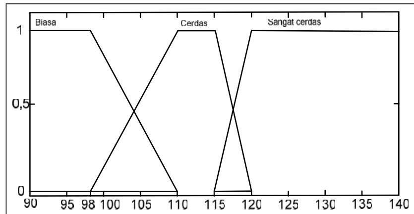
Gambar 4.6. Grafik IQ
